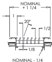
LS 1/2 20° Y FRAME
