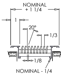
LS 1/3 20° Y FRAME
